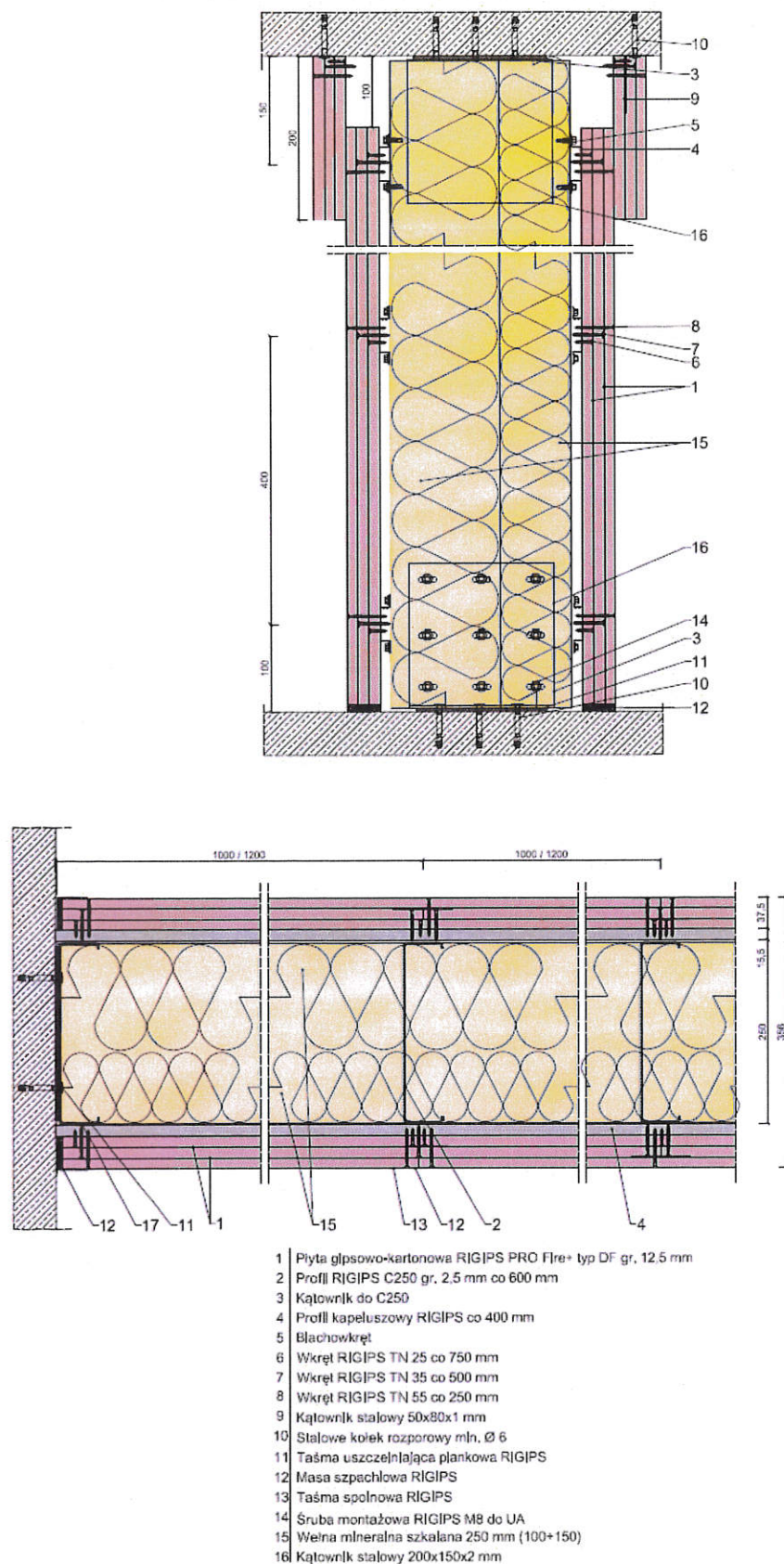
Rys. 1. Przekroje ściany systemu 3.40.14 przy opływowaniu 3x12,5 mm
