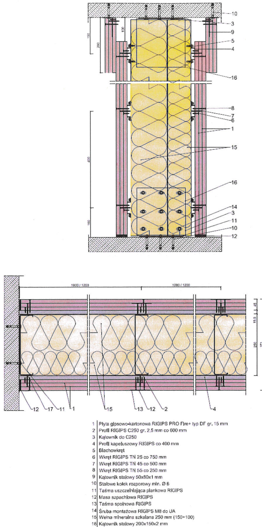
Rys. 2. Przekroje ściany systemu 3.40.14 przy opływowaniu 3x15 mm
