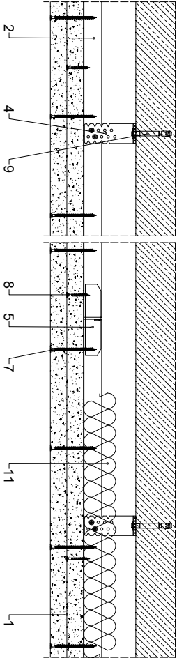
Przekrój podłużny
