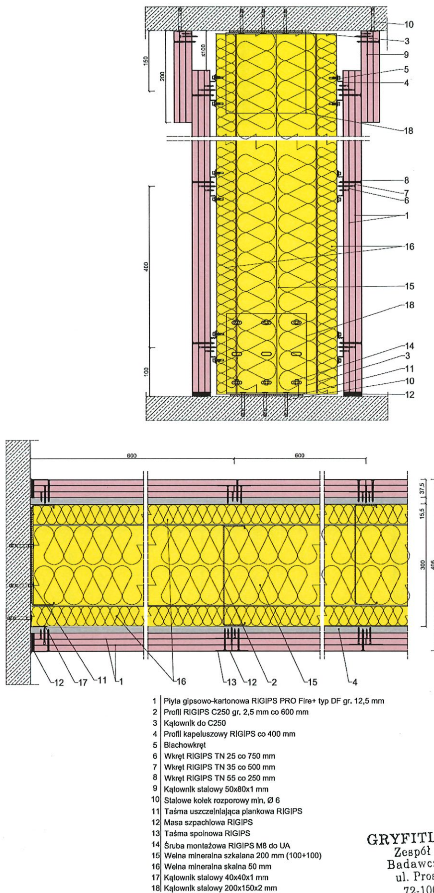
Rys. 1. Przekroje ściany systemu Rigips 3.40.14 przy opływowaniu 3x12,5 mm
