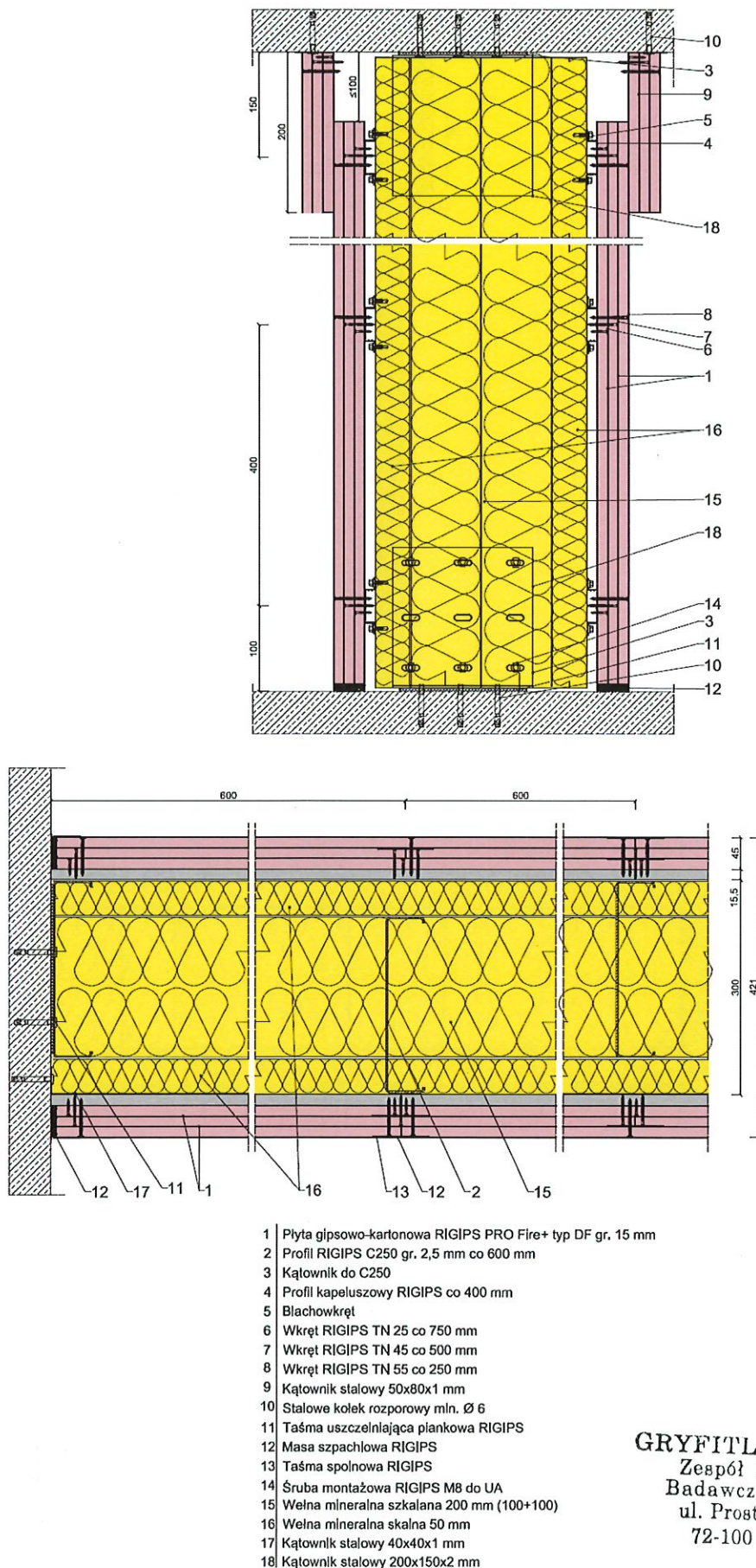
Rys. 2. Przekroje ściany systemu Rigips 3.40.14 przy opływowaniu 3x15 mm
