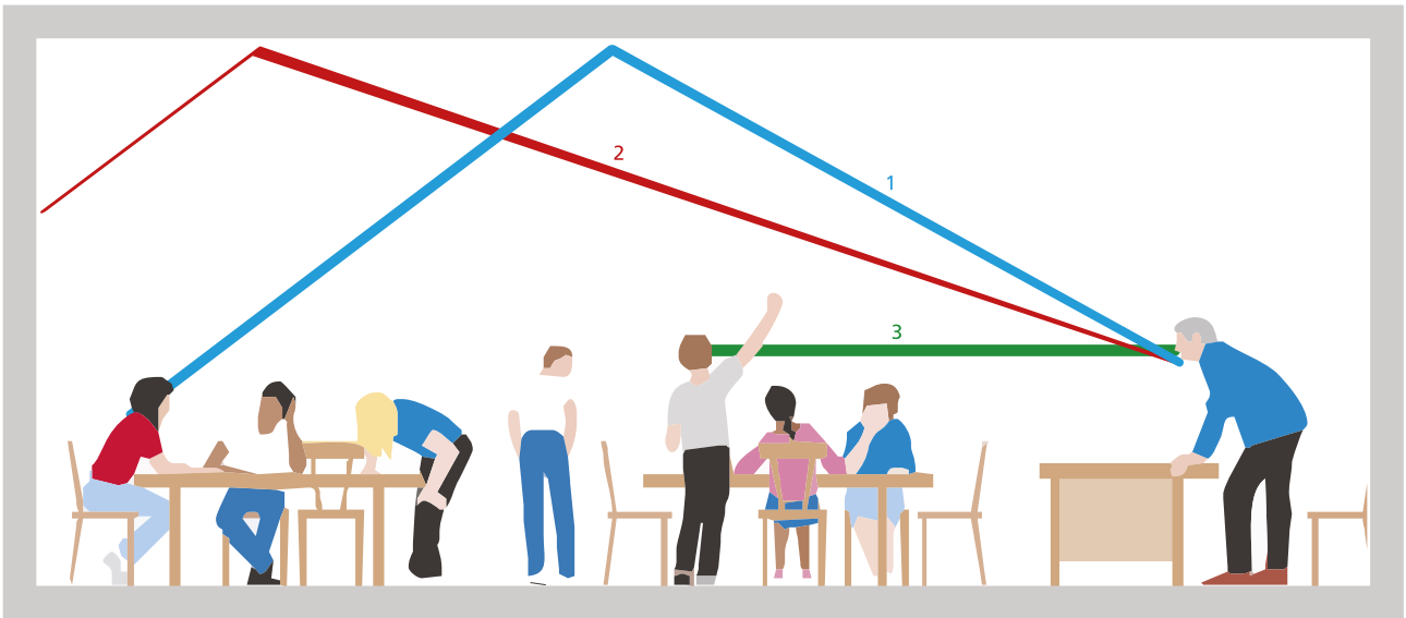
Rysunek nr 4. Schemat ideowy zjawiska absorpcji i odbicia dźwięków od urządzeń budowlanych:
