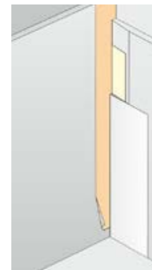
Narożne połączenie płyt gipsowo-kartonowych z powierzchnią tynkowaną: przy połączeniu z tynkiem lub betonem, przed zaszpachlowaniem, należy nakleić taśmę samoprzylepną RIGIPS PRO do połączeń ślizgowych. Po szpachlowaniu należy usunąć wystającą część taśmy.
