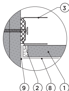
Połączenie ślizgowe
