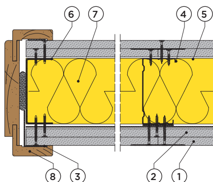
Montaż drzwi.
