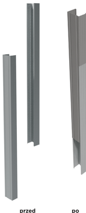
Przedłużanie profili CW „profil w profil”
