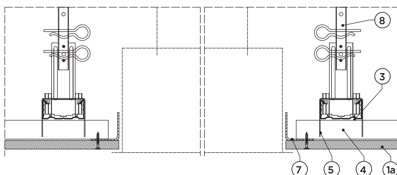
Przekrój poprzeczny
