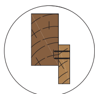
Mocowanie łaty do krokwi - widok poprzeczny
