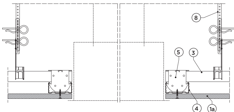
Przekrój poprzeczny
