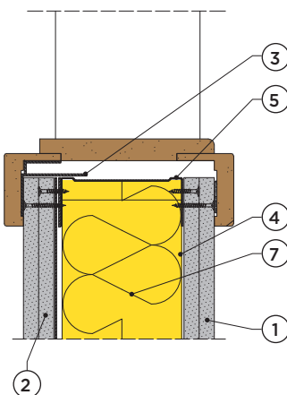
Montaż naświetla.
