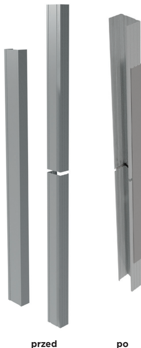
Przedłużanie profili CW na nakładkę z profilu UW
