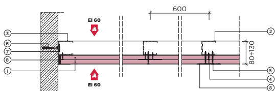
Wariant (I) układ jednościenny
