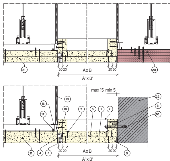
5.46.041 Przeciwpowozarowa sufitowa klapa rewizyjna RIGIPS (EI 120).
