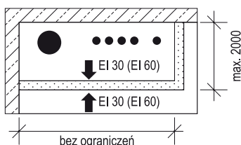
Wariant (L) układ dwuścienny
