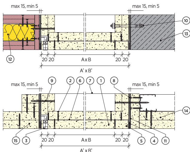
5.46.04 Przeciwpowozarowa ścienna klapa rewizyjna RIGIPS (EI 120).
