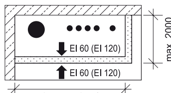
Wariant (L) układ dwuścienny
