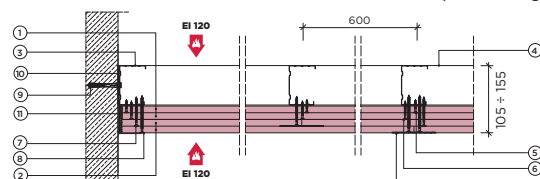
Wariant (L) układ dwuścienny
