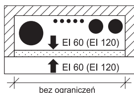
Wariant (I) układ jednościenny
