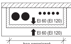
Wariant (U) układ trójsścienny
